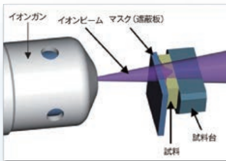
断面ミリング加工模式図
