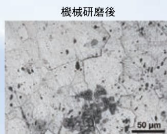
試料：鋼材
