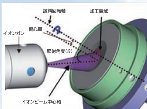
フラットミリング ® 加工模式図
