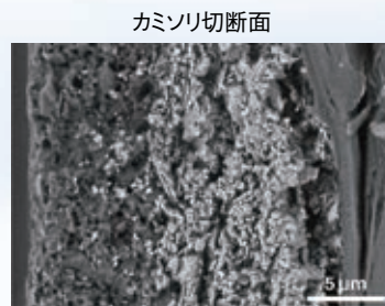
試料：感熱紙
